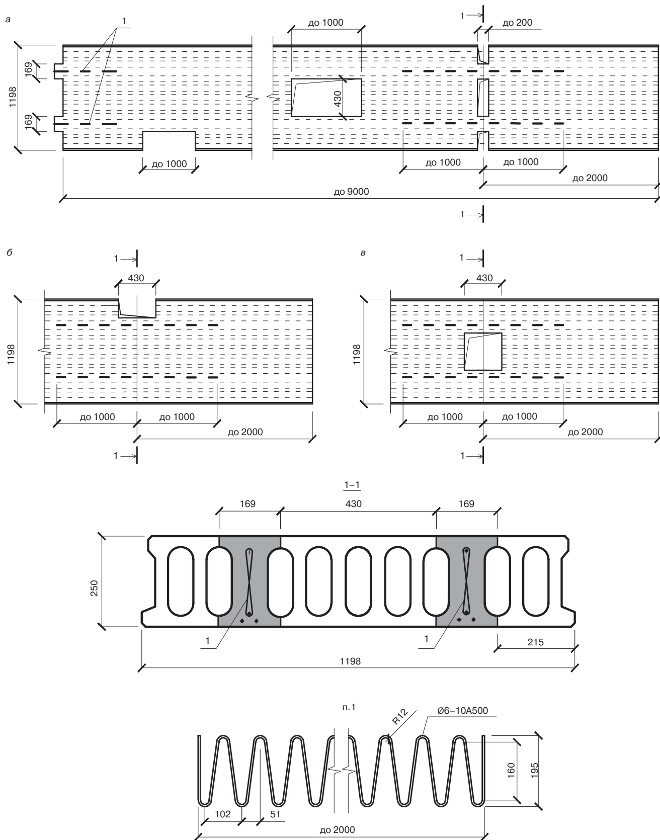
Рис. 1. Плита пустотная с многоядерными усилителями. Варианты: а – для панельных зданий; б–в – для каркасных зданий. Затененная часть плиты на сечении 1–1 обеспечивает несущую способность на полезную нагрузку 8 кПа; консольная часть плиты (до 2 м) выдерживает нагрузку от навесных стен и ограждений до 11 кН/п.м
