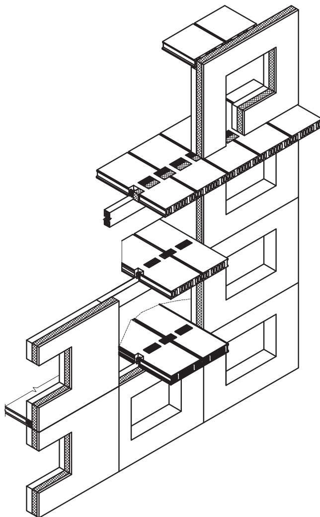
Рис. 3. Плита пустотная с многоядерными усилителями в панельном здании
