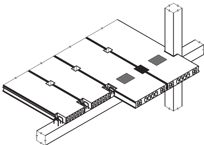
Рис. 2. Плита пустотная с многоядерными усилителями в каркасном здании
